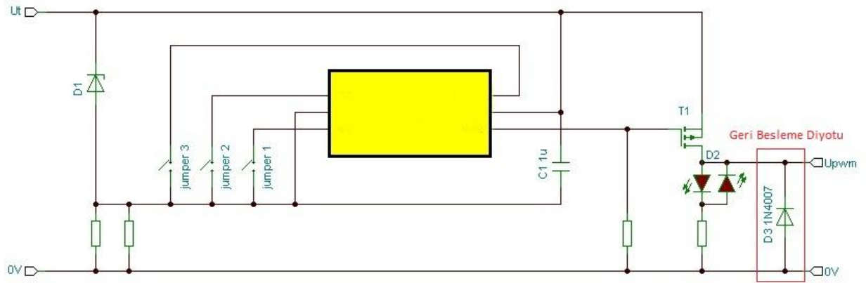
Şekil 8. PWM soket devre şemasında koruma diyotu
