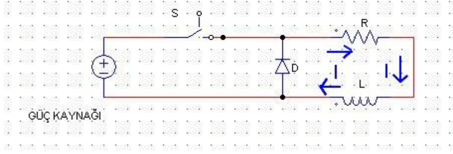
Şekil 6. Geri besleme diyotu kullanıldığında endüktansın enerjisini boşaltması
