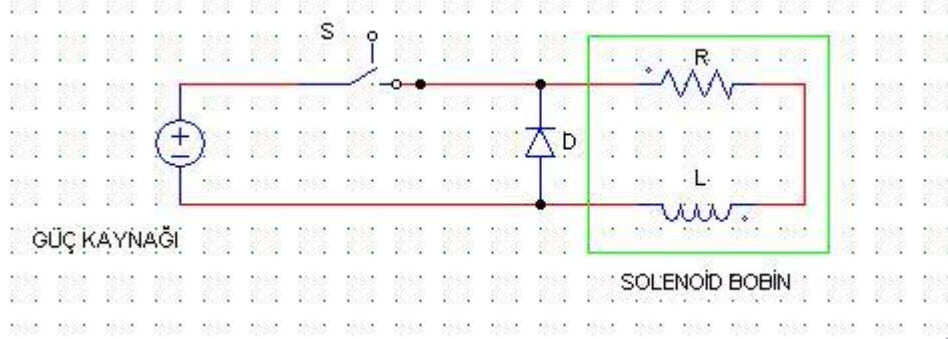
Şekil 4. Gerilim kaynağına bağlanmış ve geri besleme diyotu (D) kullanılmış solenoid bobin.
